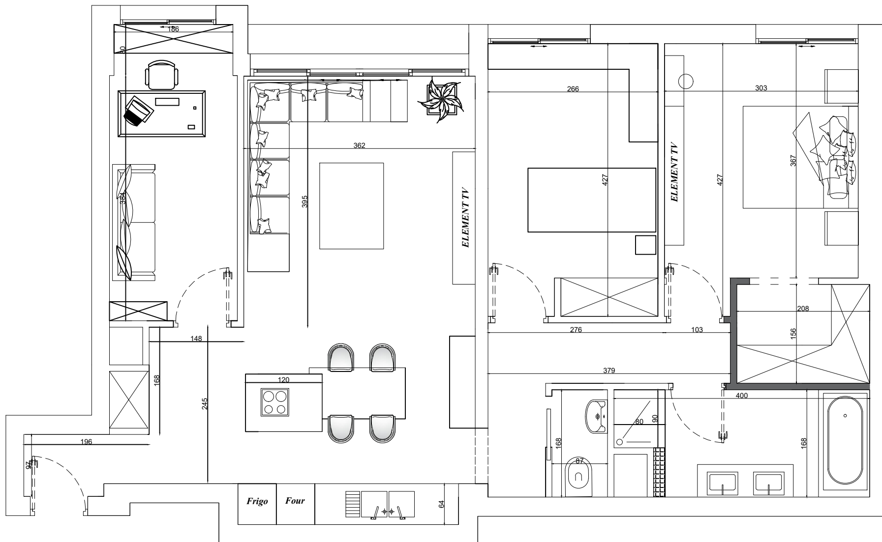
Plan Aménage
