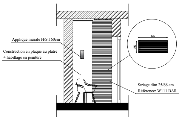
Coupe élévation A-A
