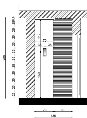
Coupe élévation A-A
