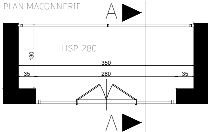
PLAN MAÇONNERIE
