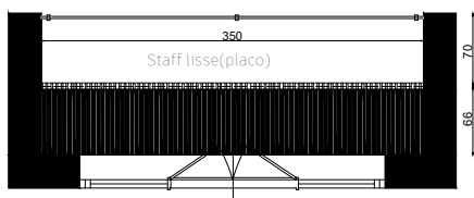
PLAN FAUX PLAFOND
